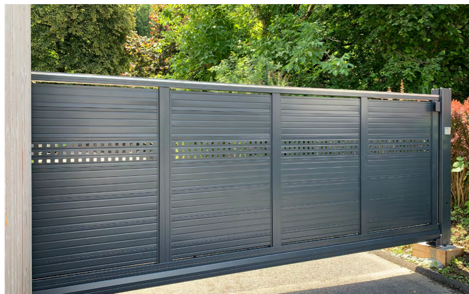
Klizna vrata Glatki lim s perforiranom trakom, antracit boja
